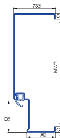
Blockzarge Typ 1
