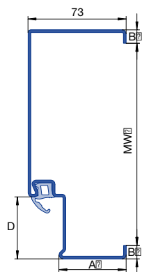
Umfassungszarge B73
